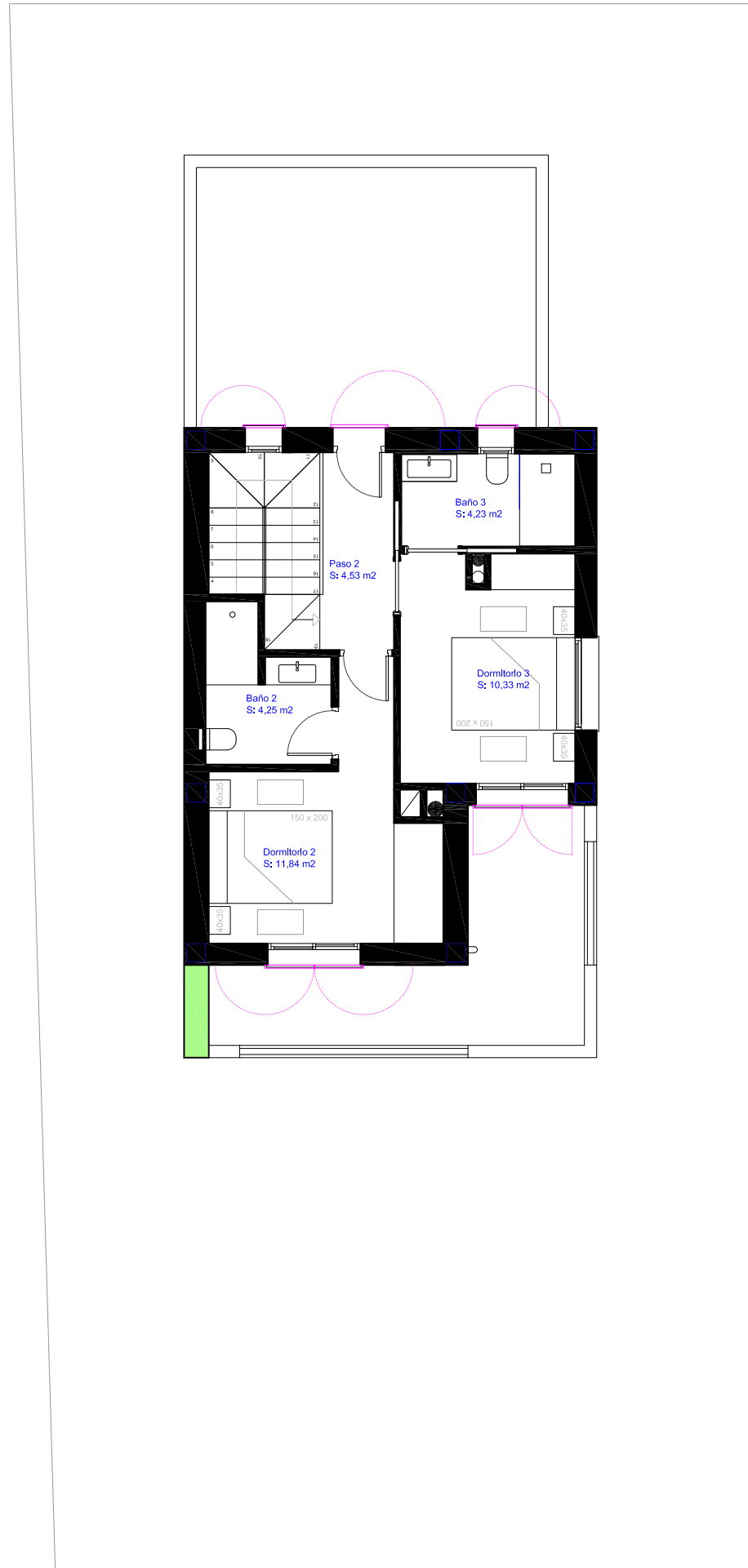
Planta 1
