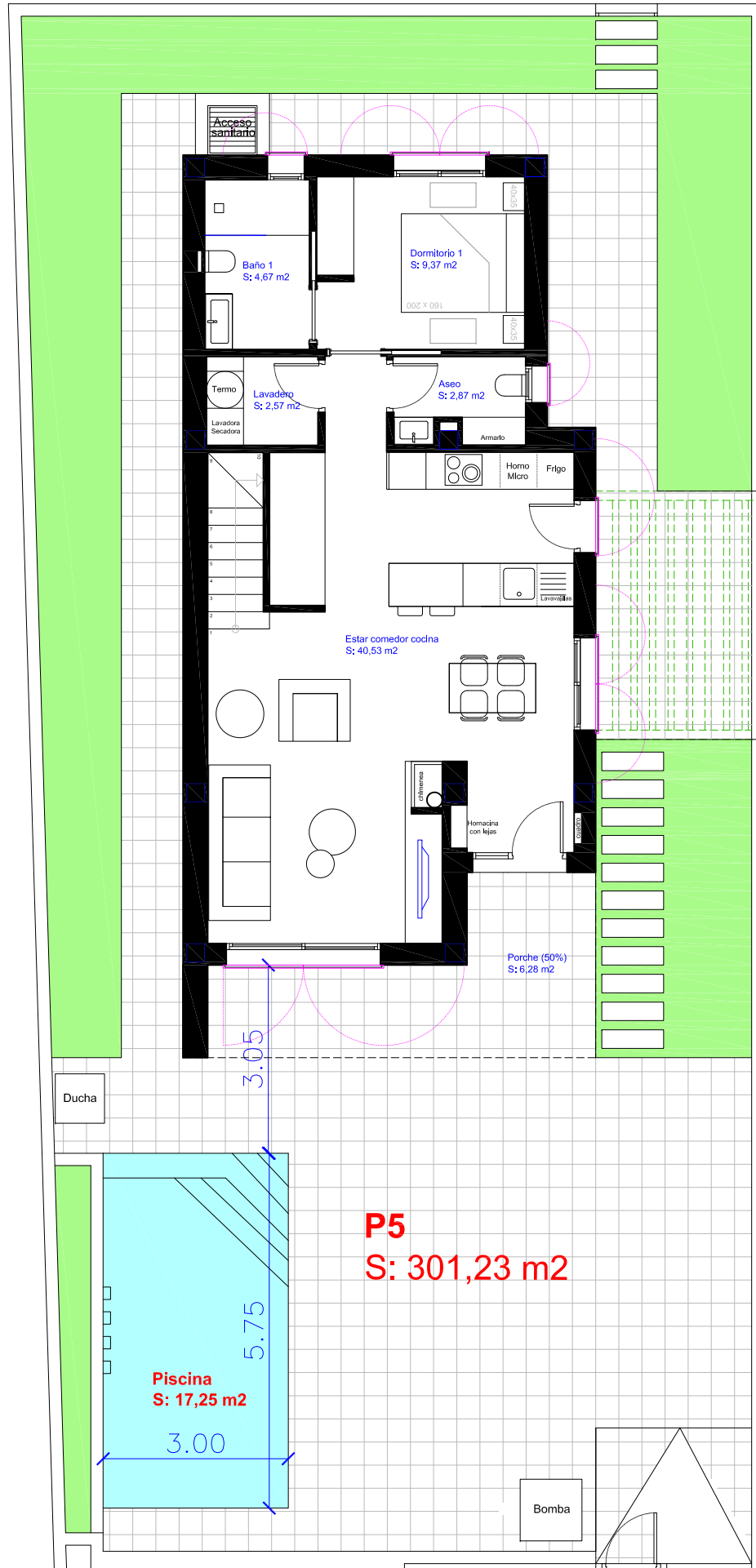
Planta baja
